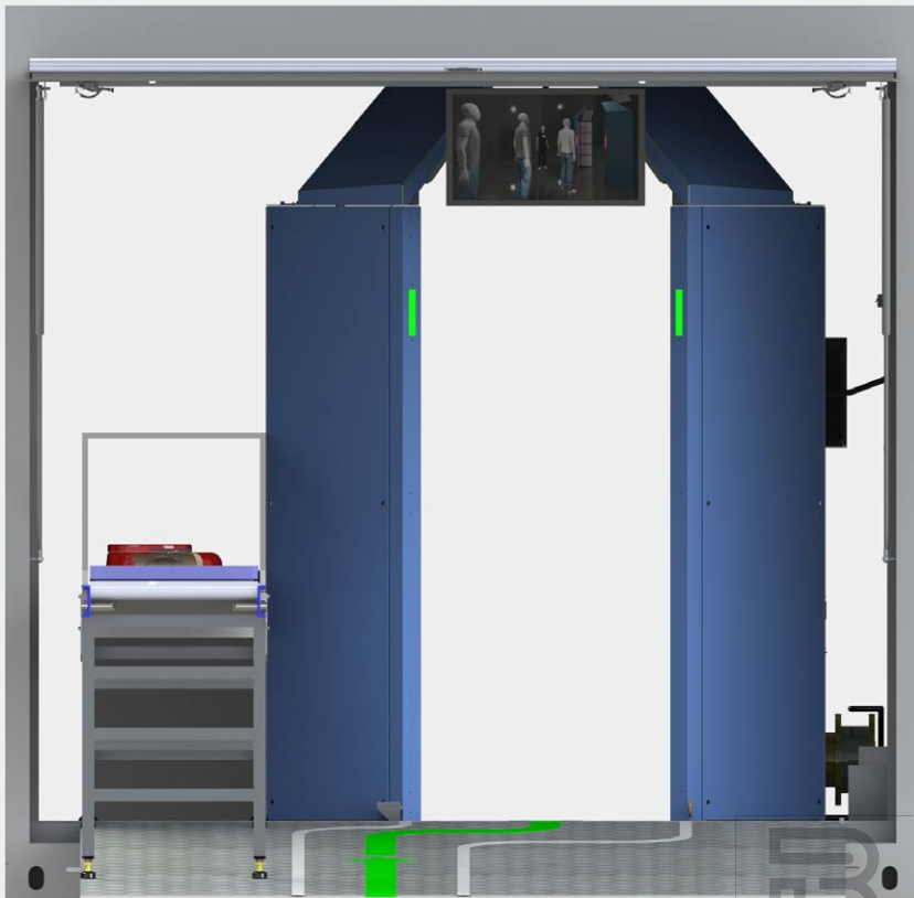
Fig.1 Illustration 3D - Vue côté entrée module déployé
