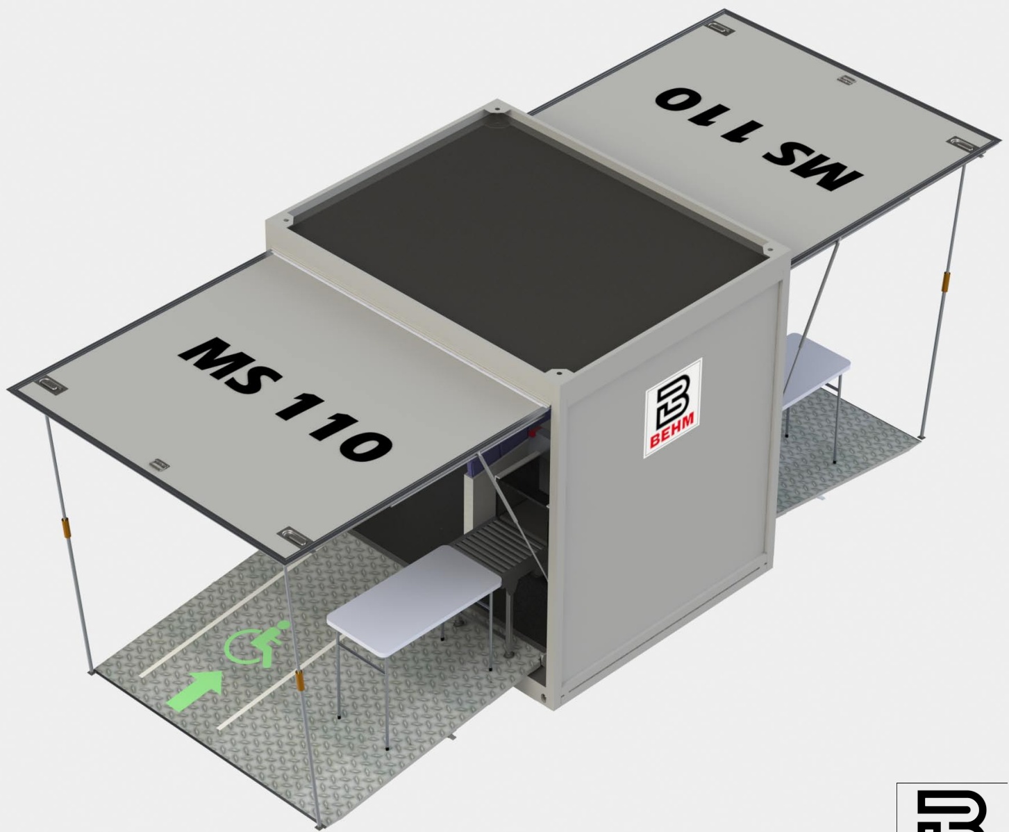
Fig.2 Illustration 3D - Vue isométrique module déployé
