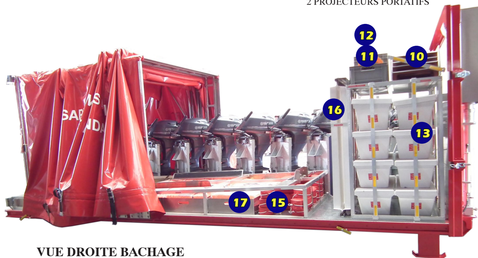
2 CAISSES iso 600*400*320 8 HELICES DE RECHANGE 2 RALONGES DE 20M TYPE DS1 1 RALLONGES DE 10 M 2 PROJECTEURS PORTATIFS
